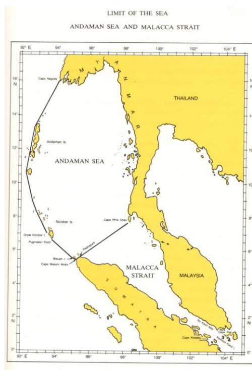
ภาพที่ 2 ขอบเขตของทะเลอันดามัน (Andaman Sea) และช่องแคบมะละกา (Malacca Strait) ( ที่มา : คู่มือการสร้างแผนที่เดินเรือ กรมอุทกศาสตร์ )
