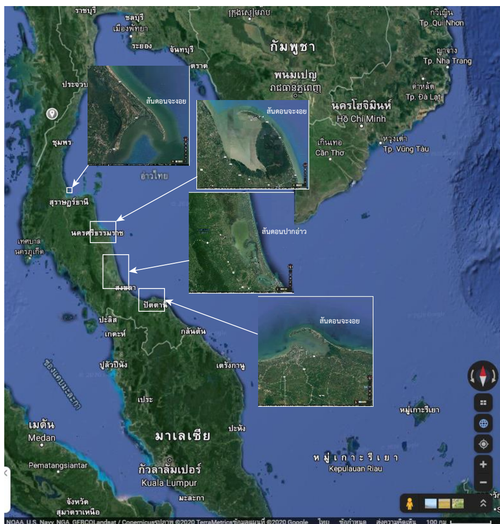
ภาพ 3.10 สันทรายขนาดใหญ่ที่เกิดจากกระแสน้ำและคลื่นพัดพาเอาทรายมาตกทับถมมีชื่อเรียกแตกต่างกันไปตามลักษณะรูปร่าง เช่น สันดอนจะงอย (Hook spit or curved spit) และ สันดอนปากอ่าว (Baymouth bar) (Google.com/maps, 2020)
