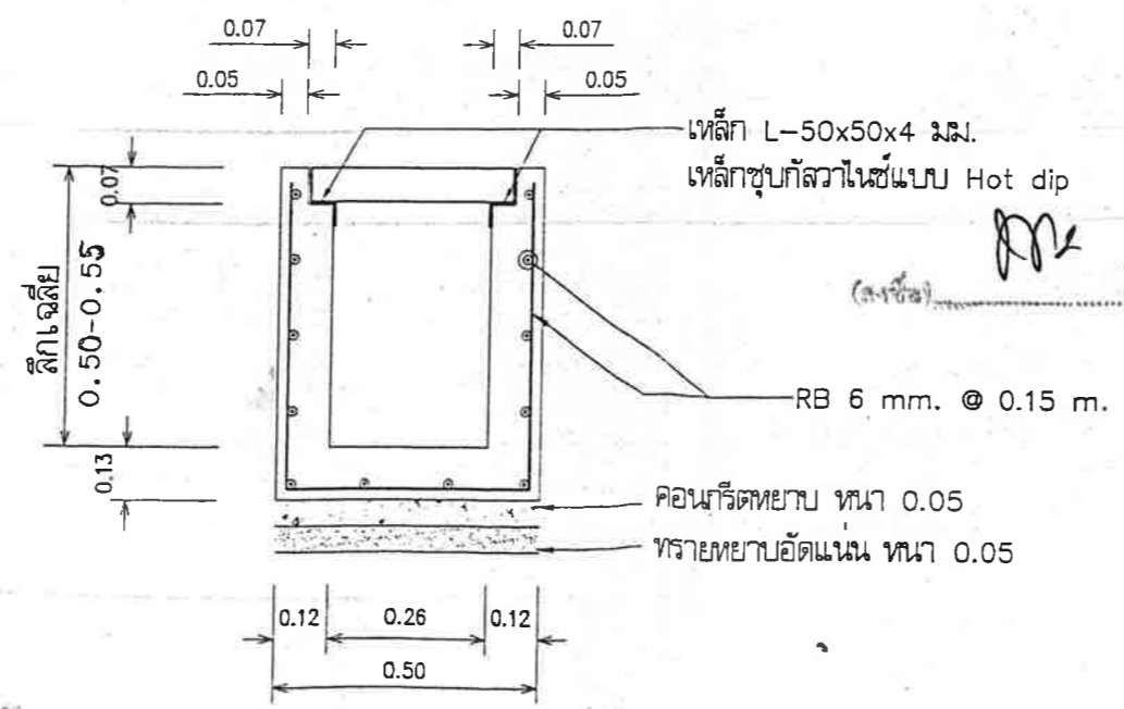
แบบขยายรางระบายน้ำ คสล.
