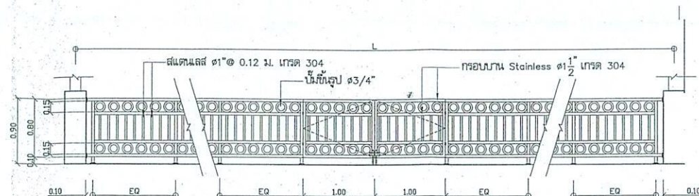
แบบขยายประตูสแตนเลส (D)
