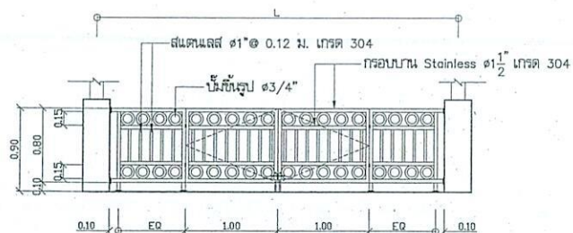
แบบขยายประตูคูลแดนเลส D1
