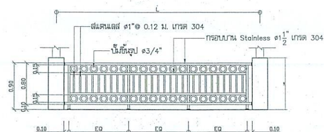
แบบขยายรั้วสแตนเลส (F)
