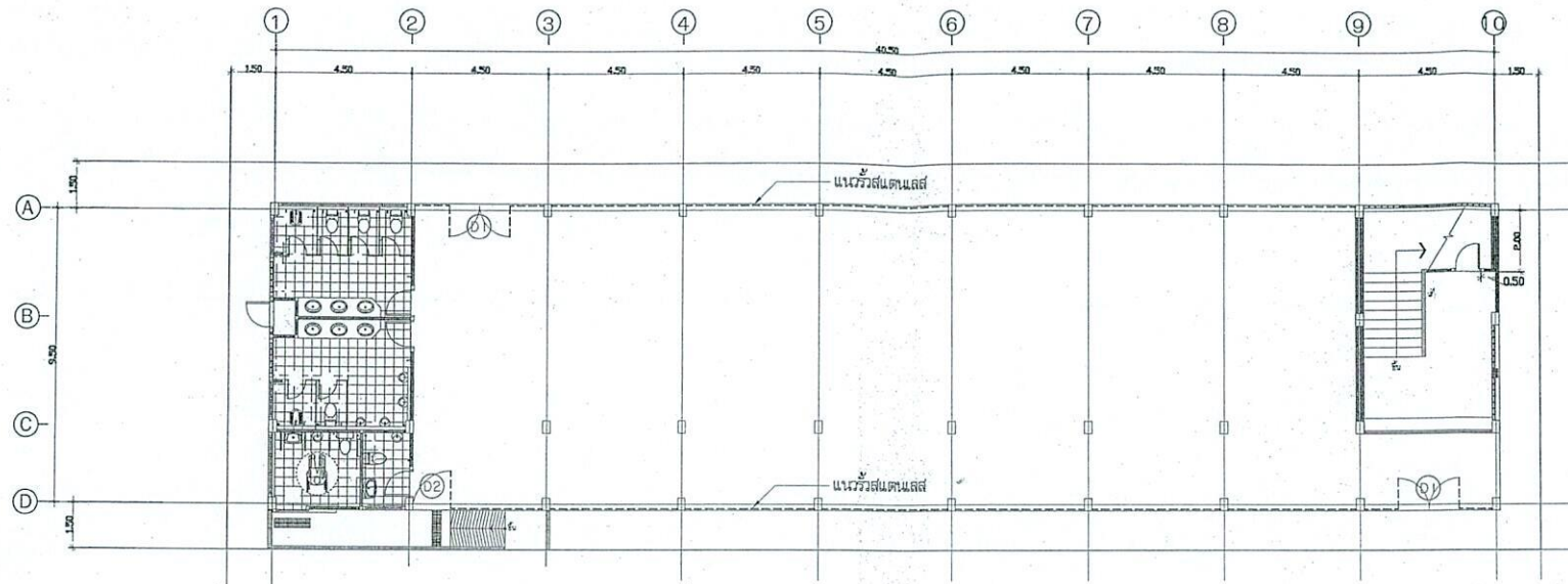
แปลนแนววีลัดแดนเลส (อาคารเรียน 7)
