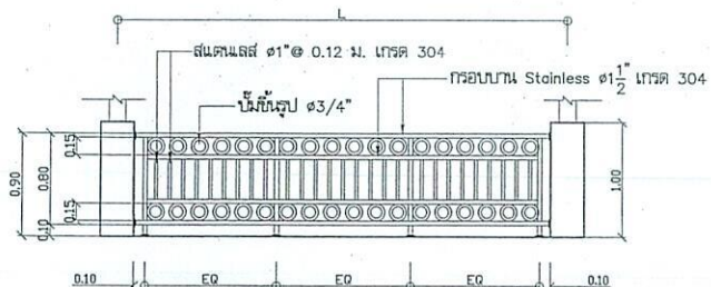
แบบขยายวีลัดแดนเลส D3
