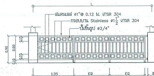
แบบขยายประตูคูลแดนเลส D2
